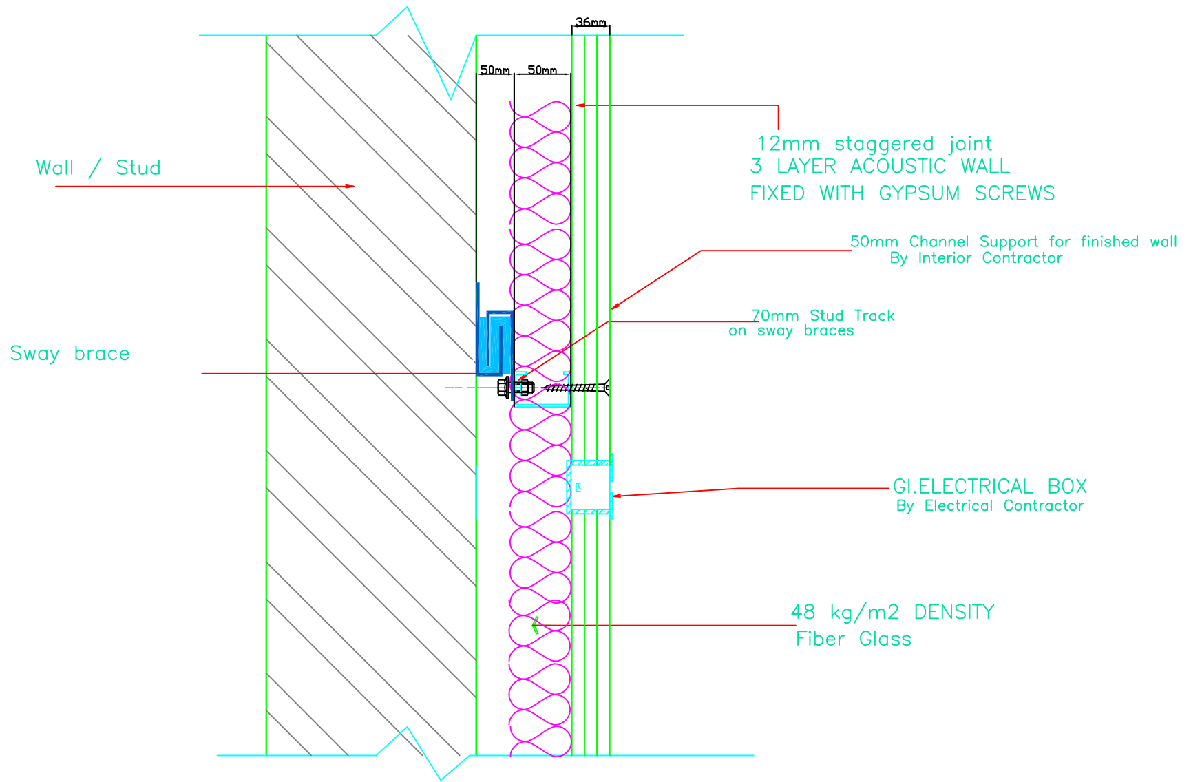
FLOATING WALL DETAILS A (N.T.S)
